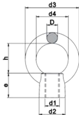
JIS 1169 Eye Nut
